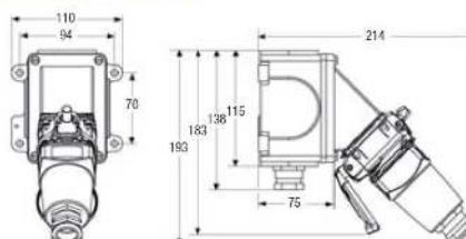
Fiche enclenchée (A1) / déclenchée (A0) dans un socle mural (45°)
